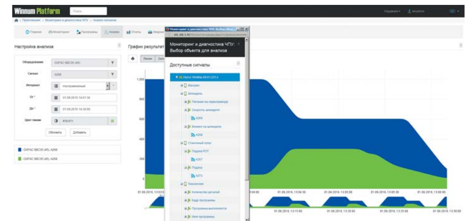
РИС. 4. ▼ Анализ параметров скорости вращения шпинделя и нагрузки
